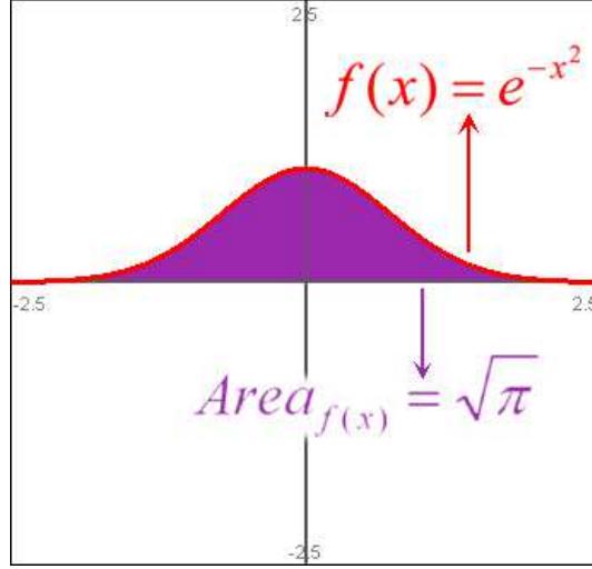
Figura 23: Ilustração para \int_{-\infty}^{+\infty} e^{-x^2} = \sqrt{\pi}.
