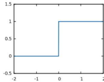
Figura 9: Esboço da função escada E = E(x) sobre [-2, 2] .
