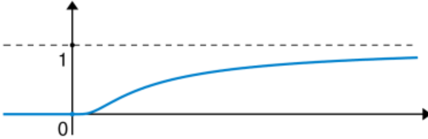
Figura 19: Gráfico de \Lambda(x) = e^{-\frac{1}{x}} , se x > 0 , com \Lambda(x) = 0 se x \leq 0 .
